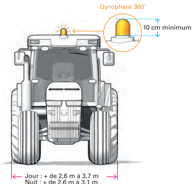
Figure 2 : un feu jaune rotatif est utilisé
