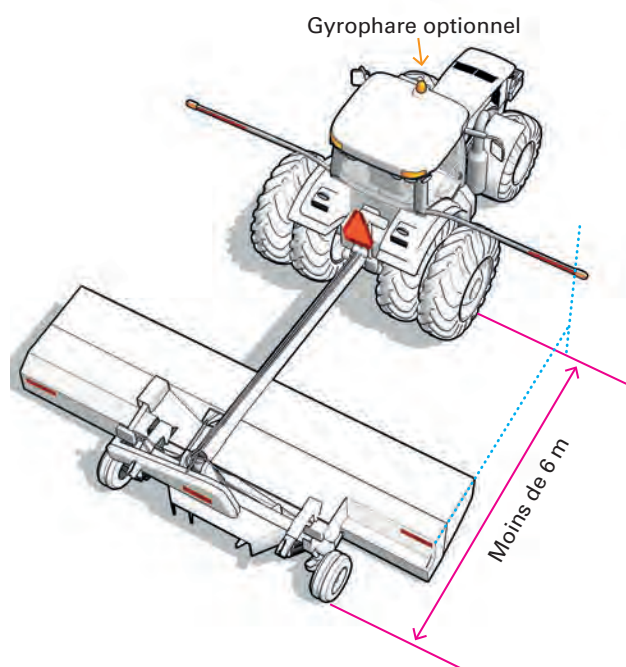
Figure 7 : distance entre les feux jaunes clignotants du tracteur et l'extrémité arrière latérale de la machine agricole remorquée.
