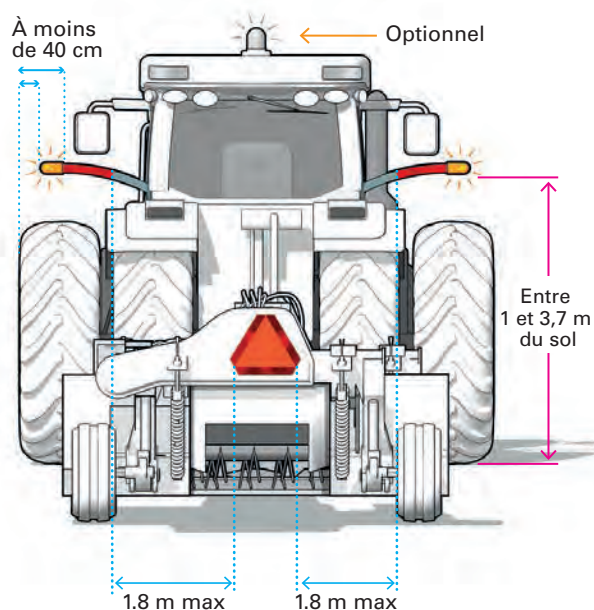
Figure 8 : Machine agricole remorquée qui n'excède pas la largeur du véhicule tracteur
