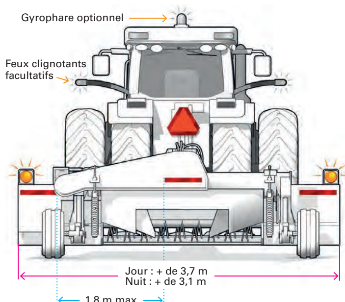
Figure 6 : machine agricole remorquée qui excède des deux côtés la largeur du tracteur qui la tire.
