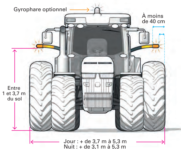
Figure 3 : bandes jaunes rétro réfléchissantes visibles de l'avant du véhicule et feux jaunes clignotants
