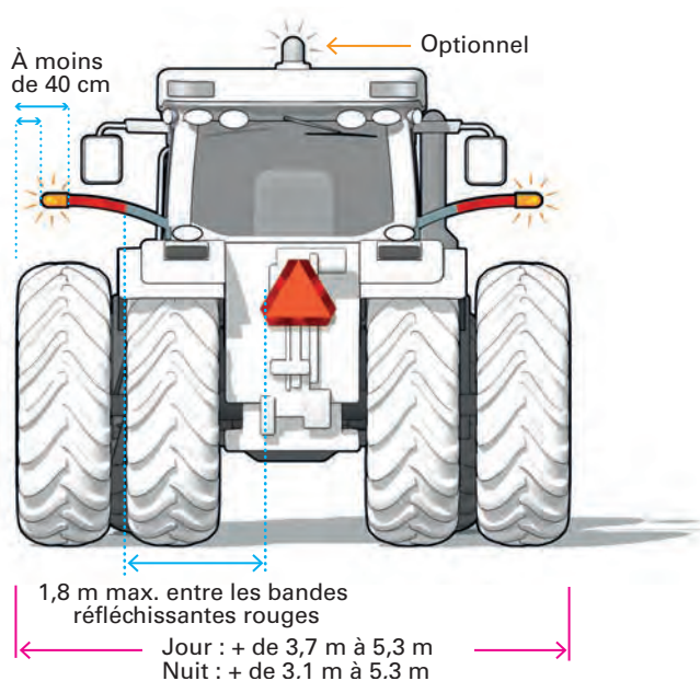
Figure 4 : bandes rouges rétro réfléchissantes et feux clignotants bidirectionnels
