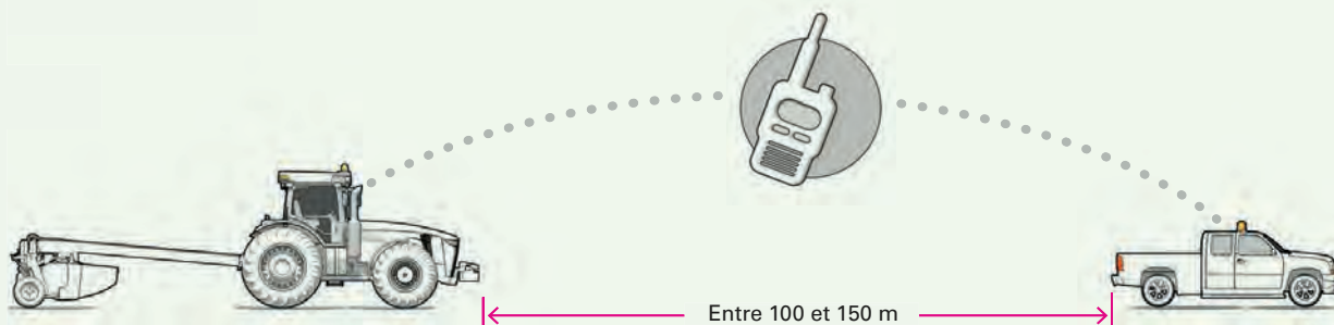
Figure 5 : véhicule d'escorte situé à une distance de 100 m à 150 m de la machine agricole ou de l'ensemble de véhicules agricoles, et muni d'un feu stroboscopique ou d'une barre de signalisation.
